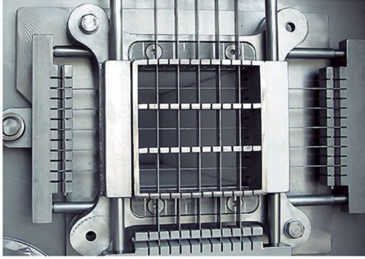
Kolay deęişebilir bıçak sistemi Easy replaceble blade system
